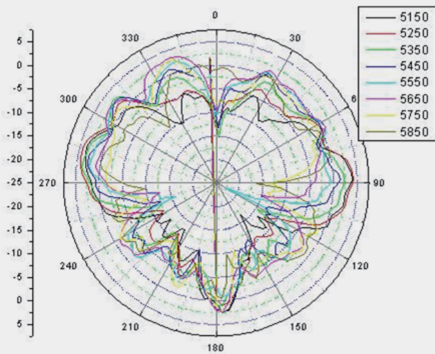
5G (PHI=0)
